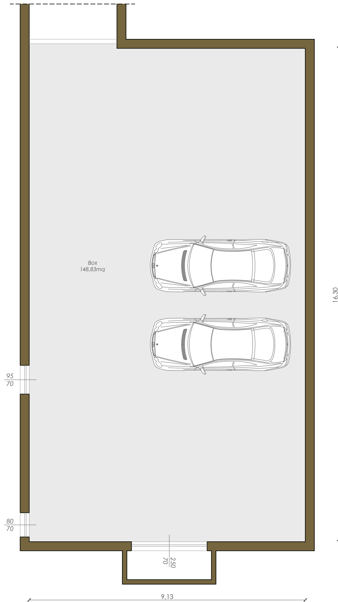
PIANTA PIANO INTERRATO
