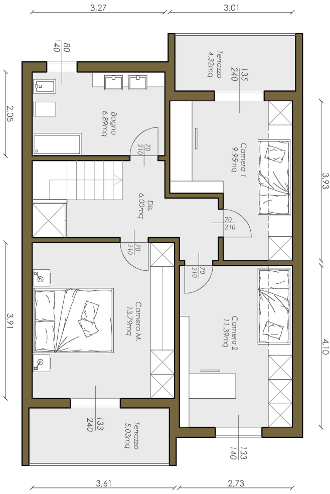
PIANTA PIANO PRIMO
